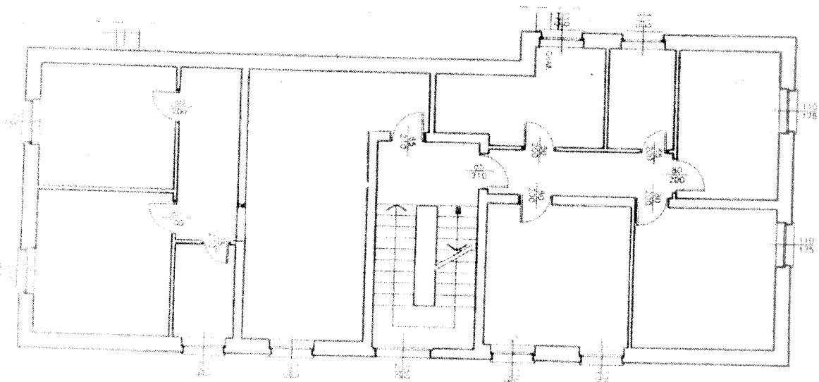
PIANO SECONDO
